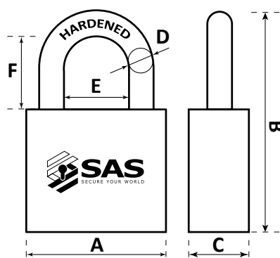
UB PADLOCKS
